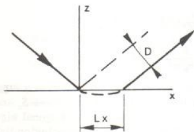
FIG. 1. The longitudinal or Goos-Hänchen shift.
